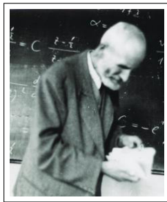
Oskar Perron 1880 – 1975
